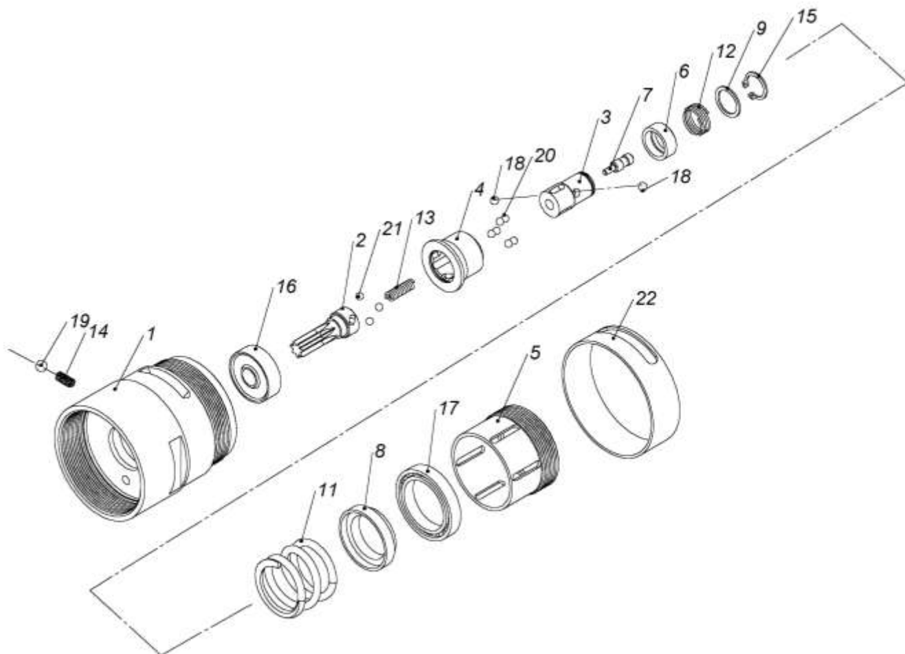
Рис. 8. Муфта предельного момента МПМ2А.62-700
